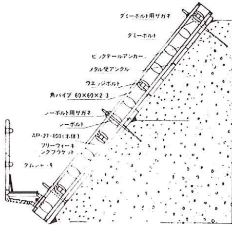
ダムフォーム図面
