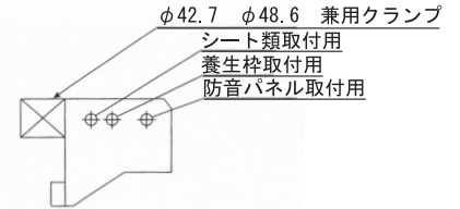
主材取付金具の穴位置
