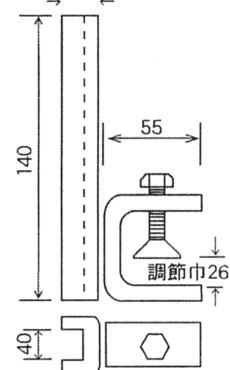
水平金具
