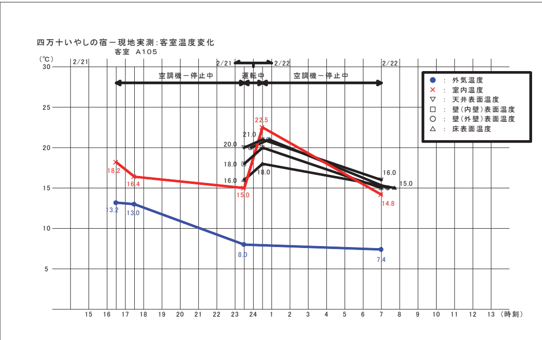
四万十いやしの宿－現地実測:客室温度変化
