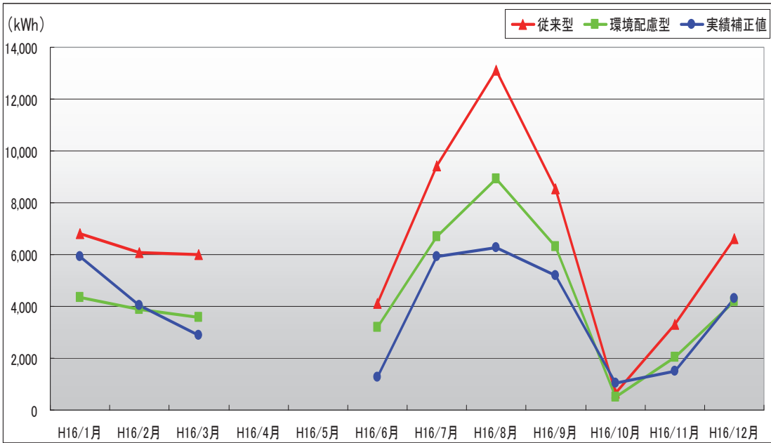
四万十いやしの宿－空調負荷低減 月別空調エネルギー使用量(電力使用量)比較
