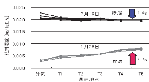
夏期と冬期のピット内湿度変化
