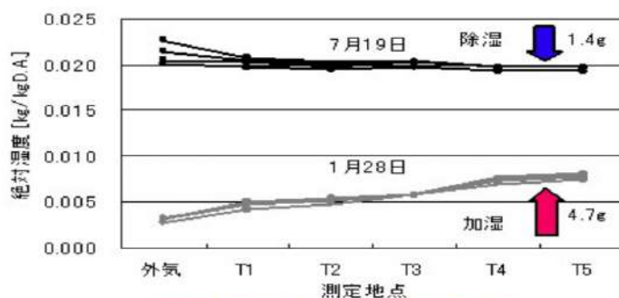
夏期と冬期のピット内湿度変化
