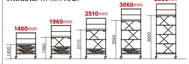
5段階調節(作業床高さ)
