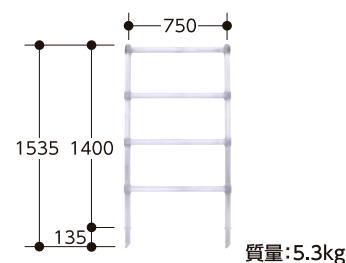
開閉式作業床 PST-KSB
