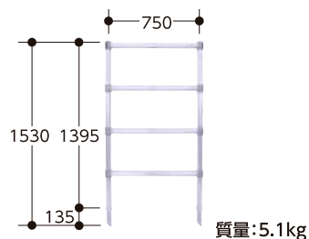
床付布枠 PST-TO
