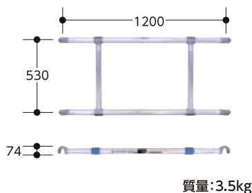
斜め連携材 PST-NR
