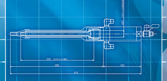
図 1:2 宇治 管構想図3 2014.07.29 U-factory H14046-K41-101
