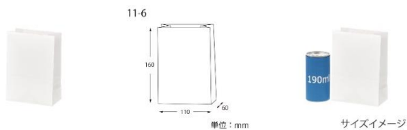
②⑤NF耐油角底袋 11-6 白無地 #004180310
