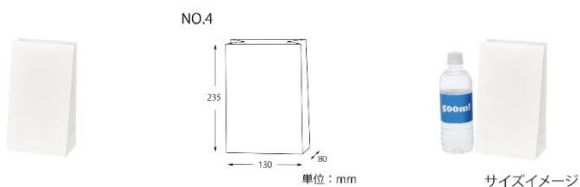
②⑨NF耐油角底袋 No. 4 白無地 #004180330
