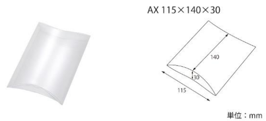
⑧クリスタルBOX AX 115×140×30 #006850014
