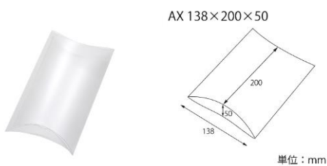
⑨クリスタルBOX AX 138×200×50 #006850015
