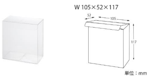
③クリスタルBOX W 105×52×117 #006850002
