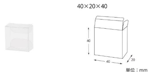
⑩クリスタルBOX V 40×20×40 #006850100
