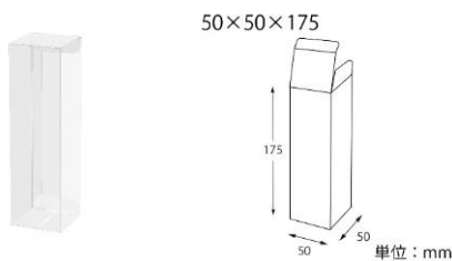
⑬クリスタルBOX V 50×50×175 #006850103
