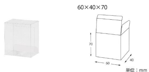
⑯クリスタルBOX V 60×40×70 #006850106
