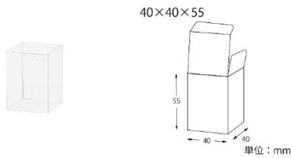
⑪クリスタルBOX V 40×40×55 #006850101
