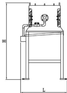
TCR-47-10型
